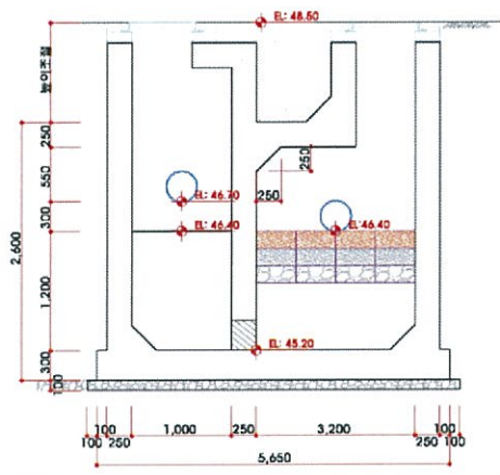
단면 A-A'
