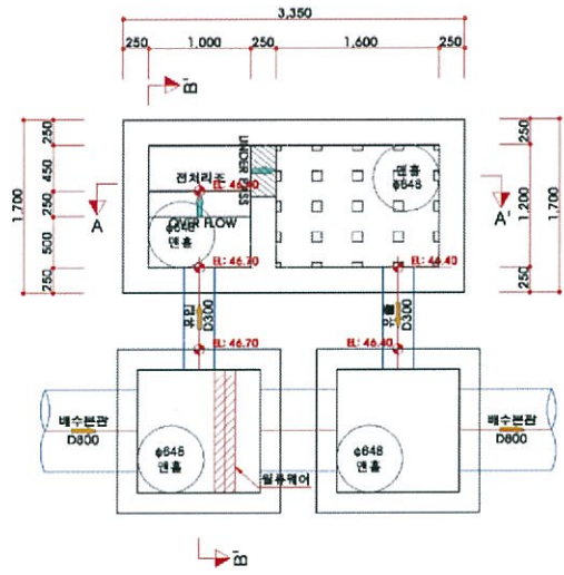
평면도
