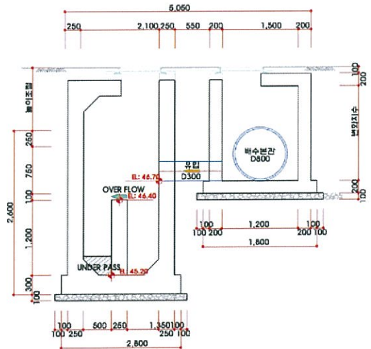
단면 B-B'
